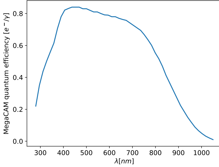
Figure 3.4 – Courbes d’efficacité quantique de MegaCAM (caméra utilisée dans le relevé SNLS), les valeurs peuvent être trouvées ici .
