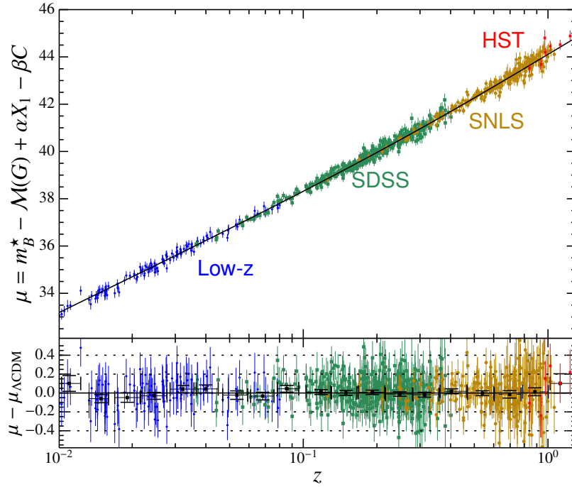
Figure 1.6 – Diagramme de Hubble de l’analyse JLA (2014). La quantité en ordonnées est le module de distance \mu = 5\log_{10}(d_L(z)/10\text{pc}) . Les résultats sont comparés au modèle \Lambda\text{CDM} . Les résidus sont présentés dans le panneau du bas, les points noirs sont les résidus moyennés par bin de redshift.
