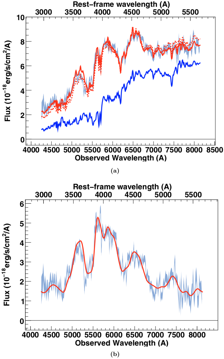
Figure 3.2 – Haut : Spectre de la supernova SNLS-06D4co ( z = 0.437 , 3.5 jours après le maximum de luminosité) mesuré avec le VLT (en gris-bleu) possédant une contamination relativement importante de la galaxie hôte. Un ajustement simultané du spectre et des courbes de lumière mesurées pour cet évènement (ligne rouge avec recalibration sur les données photométriques et tirets rouge sans) est produit en utilisant le modèle spectrophotométrique SALT2 (voir section 3.7.2.a) en considérant que le spectre est une combinaison du spectre d'une SN Ia et d'une galaxie (ligne bleue). Bas : Spectre de la SN Ia obtenu en soustrayant le modèle de galaxie (S0). Ce spectre est identifié comme celui d'une SN Ia en raison de sa compatibilité avec le modèle spectrophotométrique et de la présence d'une large absorption autour de 3800\text{\AA} dans le référentiel au repos, attribué au CaII et caractéristique des SNe Ia. Figures reproduites de BALLAND et al. (2009)
