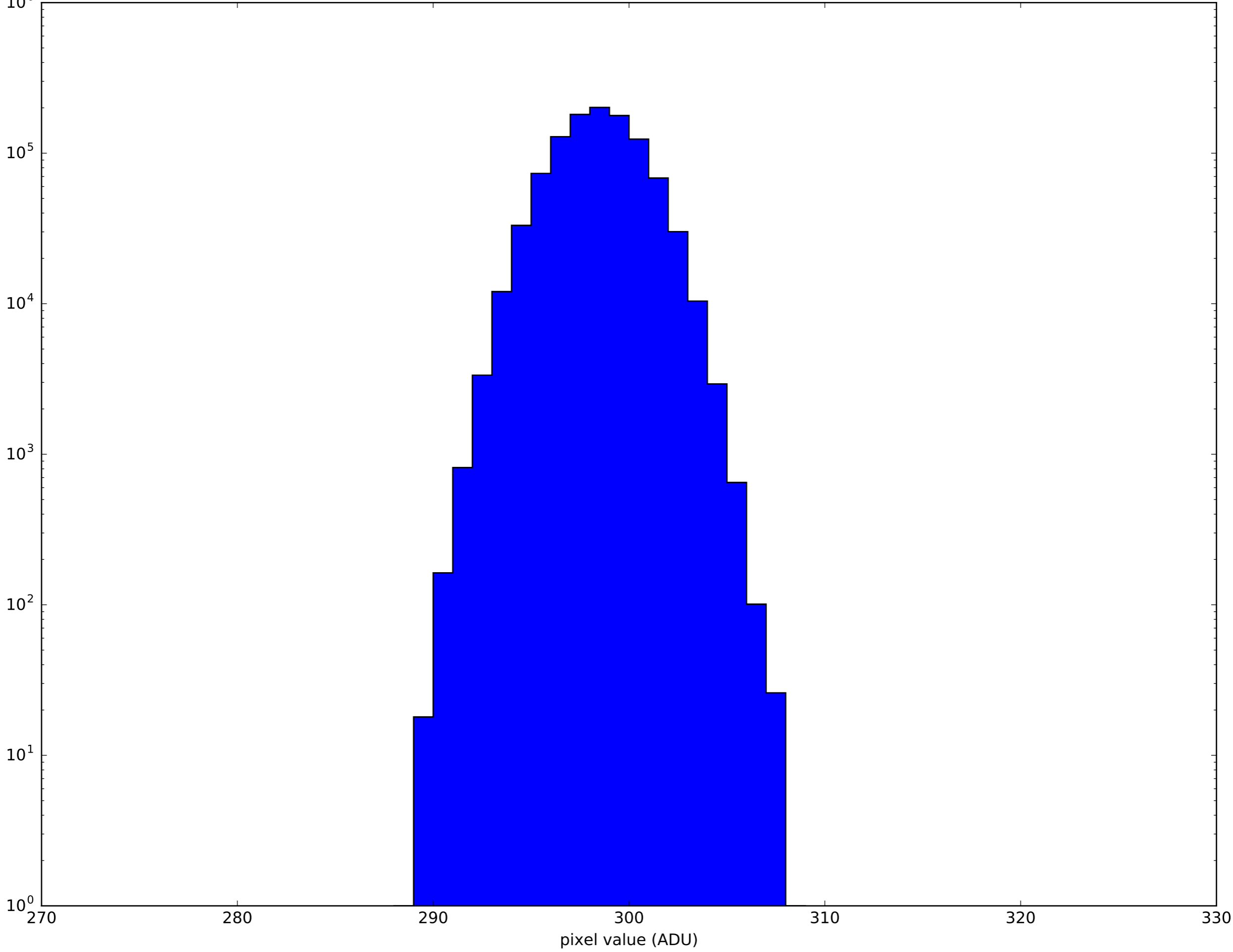
ANDOR Dark frame - exposure 500ms - readout 100MHz
