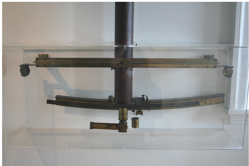
Fig. 1 – Secteur zénithal (téléscope pointant au zénith, permettant la mesure de la distance zénithale des étoiles). Conçu pour James Bradley, il est installé à l'observatoire de Greenwich. C'est avec cet instrument que J. Bradley découvrit l'aberration de la lumière et la nutation de l'axe terrestre (photos L. Le Guillou).
