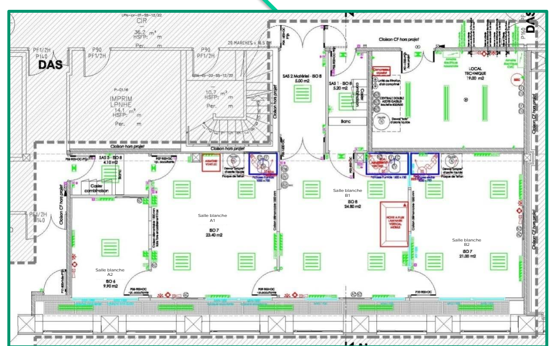
Détail salles blanches
