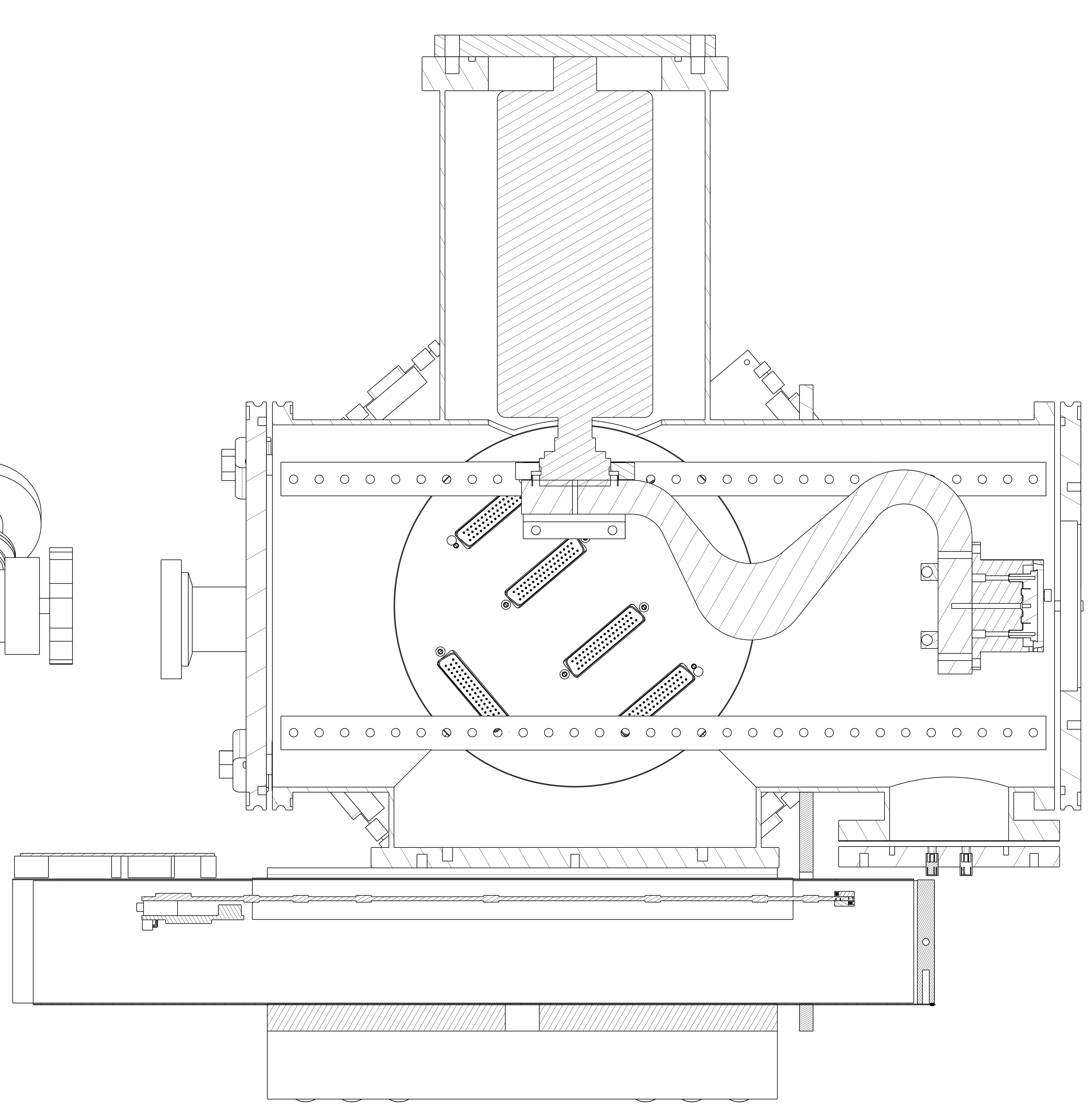
Coupe A-A Echelle : 1:1
